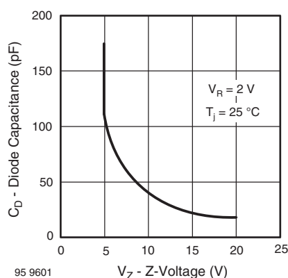
Fig. 5 - Diode Capacitance vs. Z-Voltage
